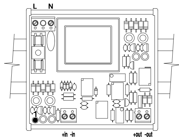
Připojovací svorky
