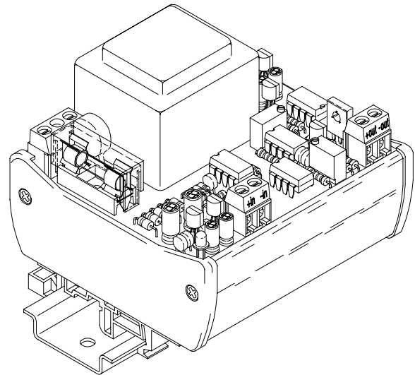
Připojovací svorky
