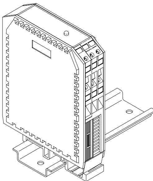
Připojovací svorky
